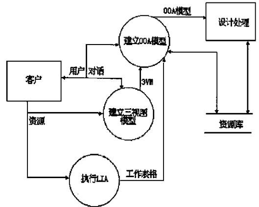
图5 发现对象技术概要
