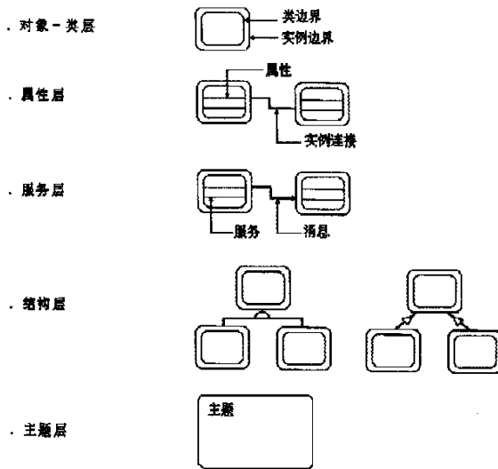
图 1 OOA 模型的结构
