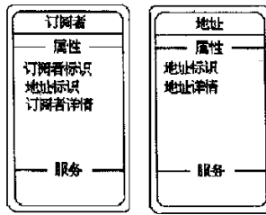
图 8 属性层(举例)
