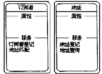
图 9 服务层(举例)
